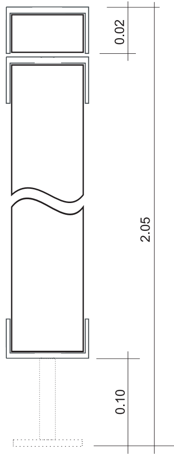
Schnitt Türe
